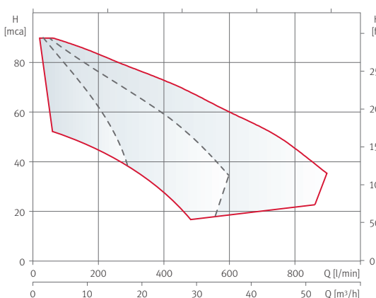
Courbes hydrauliques CPE3 à 2900 rpm
