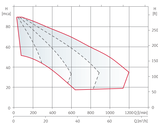
Courbes hydrauliques CPE4 à 2900 rpm
